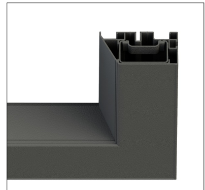
Formschönes Aluminium-Funktionsprofil von 7,5 cm Breite und 3,8 cm Tiefe
