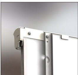
Detail des oberen Kunststoffs Klatschleiste
